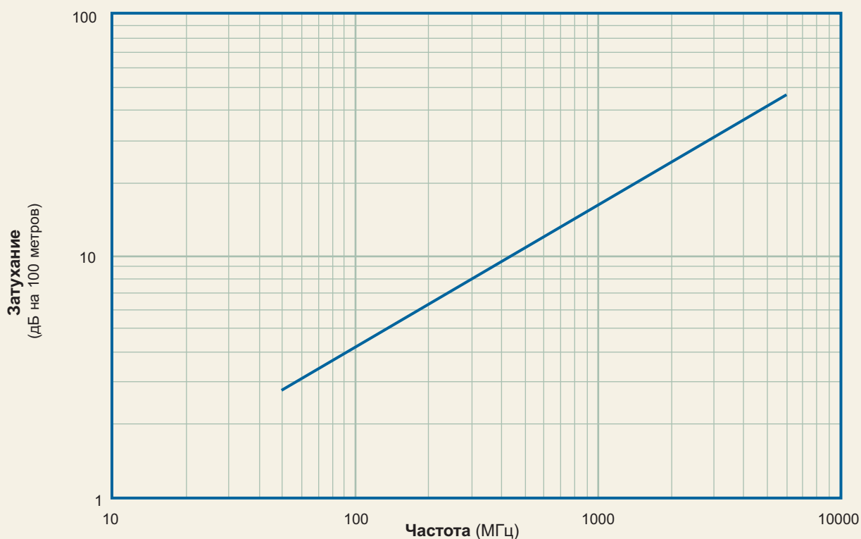
Типовое затухание 8D-FB CCA PVC
